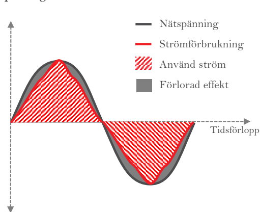
Spännings och strömkurva med PFC
