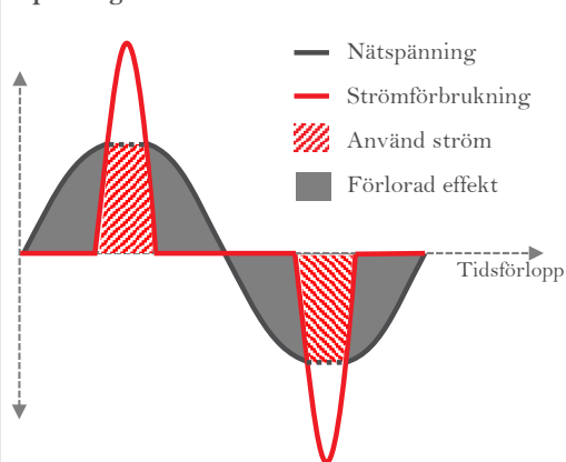
Spännings och strömkurva utan PFC
